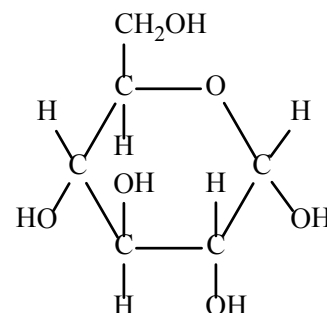
Molécula 3
