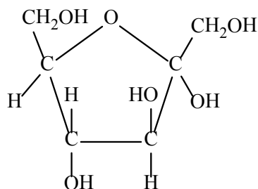
Molécula 5
