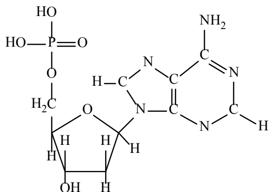
Molécula 1
