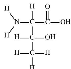
Molécula 6
